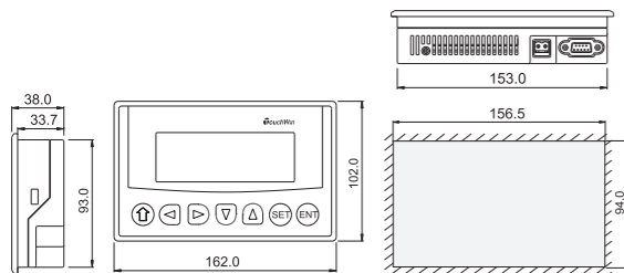
OP320/OP320-S
