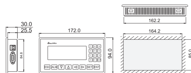
OP320-A/OP320-A-N/OP320-A-S
