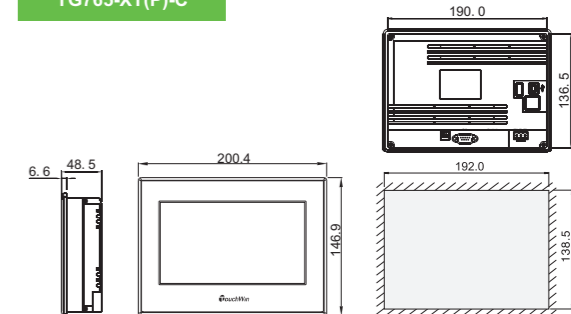
TG765-XT(P)-C
