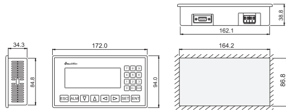
OP325-A/OP325-A-S/MP325-A/MP325-A-S
